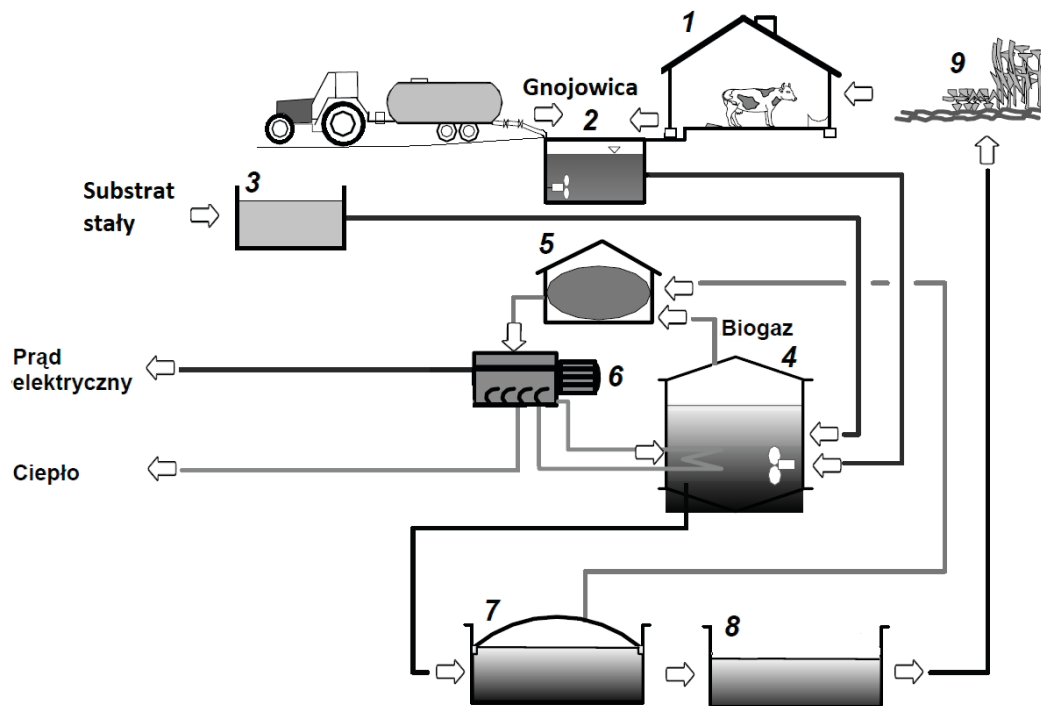
Schemat biogazowni rolniczej. 1 – obiekt inwentarski, 2 – zbiornik na gnojowicę, 3 – silos na substrat stały (np. kiszonkę), 4 – komora fermentacyjna, 5 – zbiornik na biogaz, 6 – agregat kogeneracyjny, 7 – zbiornik pofermentacyjny, 8 – zbiornik na poferment, 9 – pole uprawne
